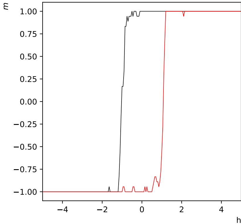
Hystérésis de l'aimantation réseau de taille L=6 - h=5 à T=1.5
