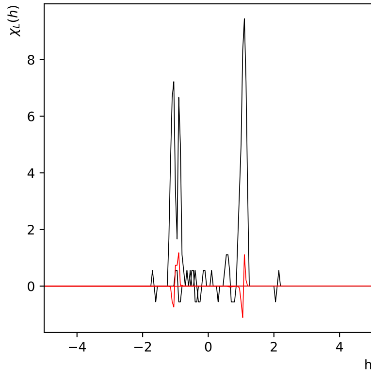
\chi_L(h) réseau de taille L=6 à T=1.5
